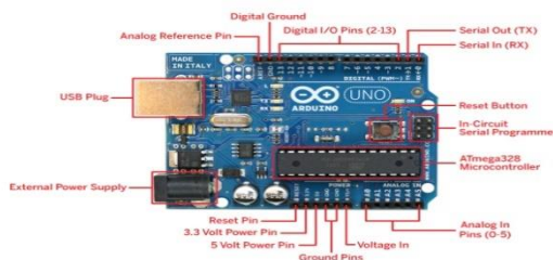
Gambar Bagian-bagian Arduino Uno
